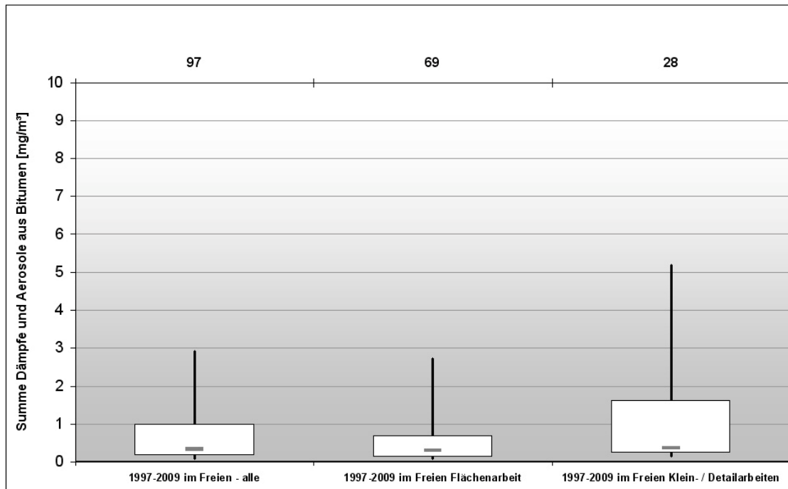
Abbildung 2A*: In Europa ermittelte Expositionen für Dämpfe und Aerosole aus Bitumen beim Schweißen von Bitumenbahnen bei Detail- bzw. großflächigen Arbeiten [ \text{mg}/\text{m}^3 ]
